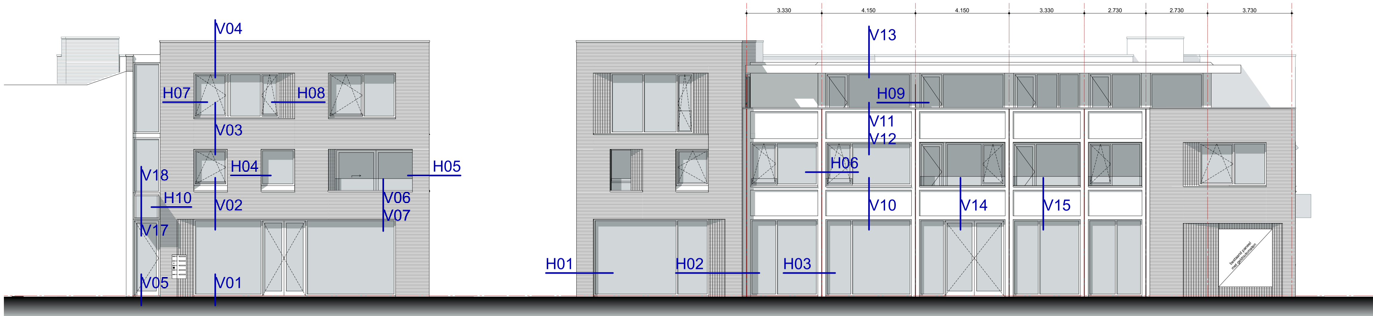
Voorgevel - Rijksstraatweg
