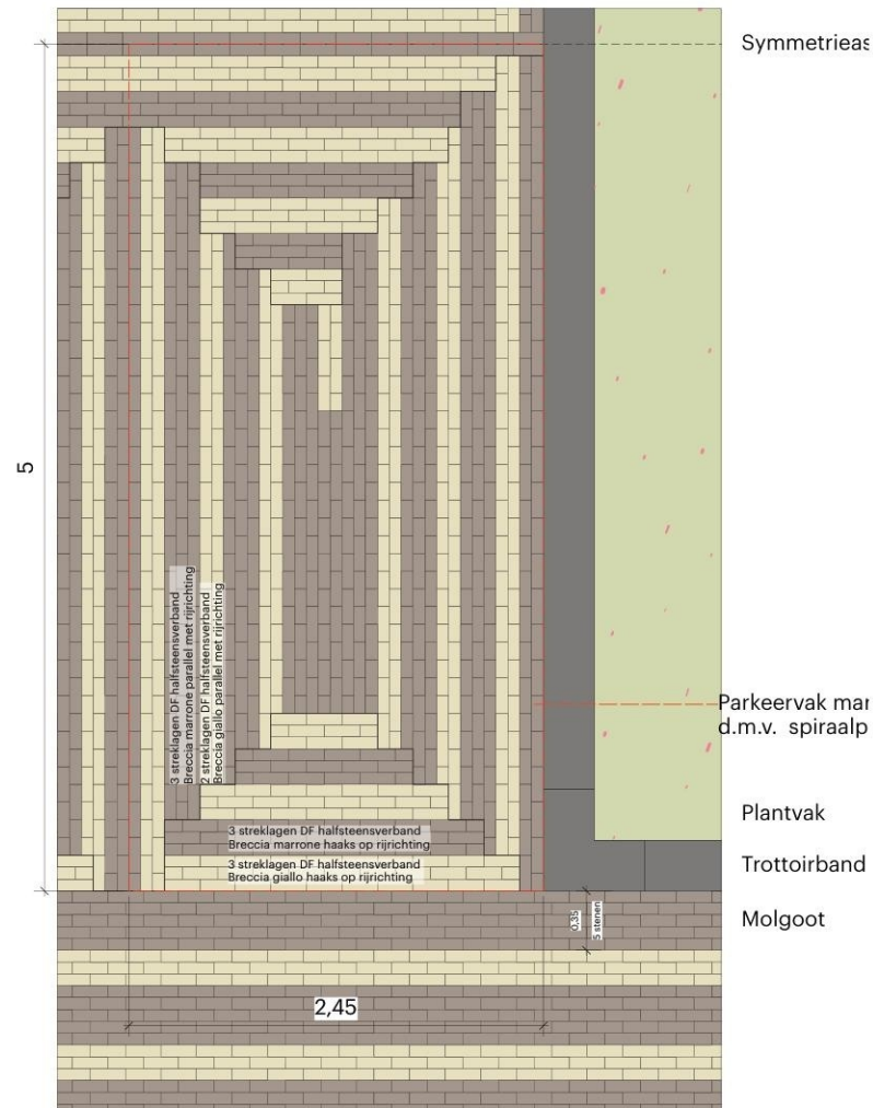
Detail 2: legpatroon parkeervak binnenplein
