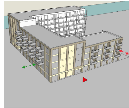
(3) Opbouw gevelindeling - toepassing buitenruimtes: - aan Antillenstraat <-> half verdiept in gevel; - aan Groenzone <-> volledig uitkragend; - aan Boulevard <-> half verdiept in gevel; opbouw van zwaar naar licht.
