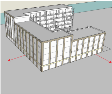
(1) Opbouw gevelindeling: - Horizontale en verticale gevelindeling door structuur van repeterende portalen; - Doorlopende horizontale band op 1e verdieping; - Alzijdig gebouw ontwerp; prominente voorgevels.
