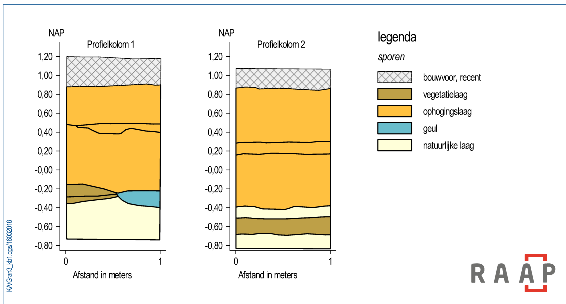
Figuur 4. Profielkolommen.
