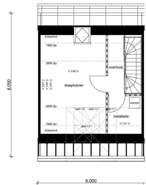
type C optie 2e verdieping kavel 1 t/m 8
