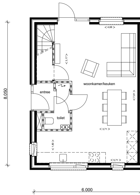
type E optie Begane grond kavel 9
