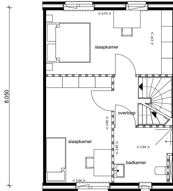
6.000 type A1 optie 1e verdieping kavel 1 t/m 8
