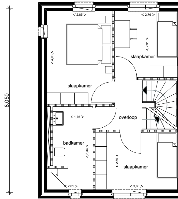
6.000 type F basis 1e verdieping kavel 9
