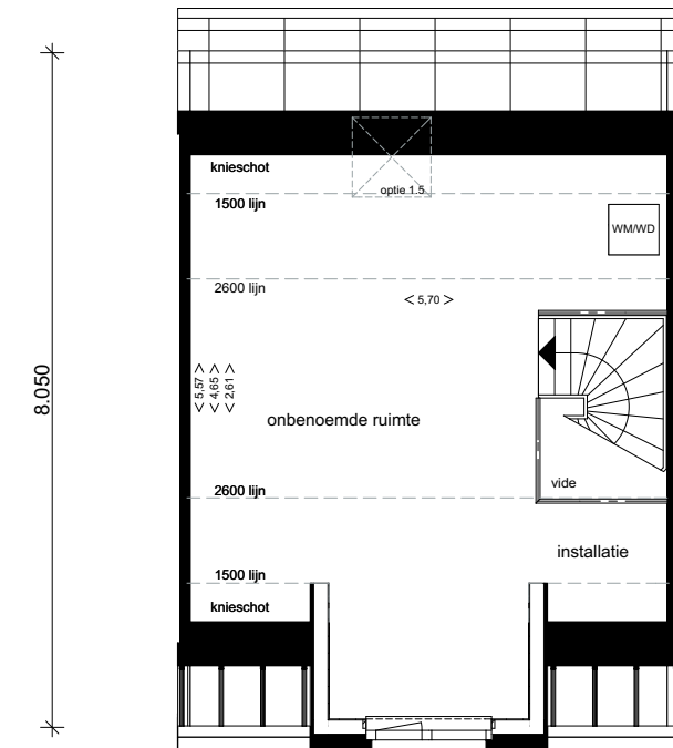
6.000 type A basis 2e verdieping kavel 3, 5 en 8 (arkeneel)
