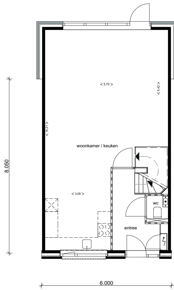
Begane grond (optie 3.3)
