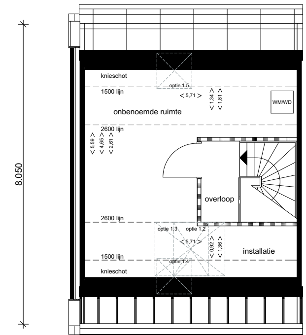
6.000 type F basis 2e verdieping kavel 9
