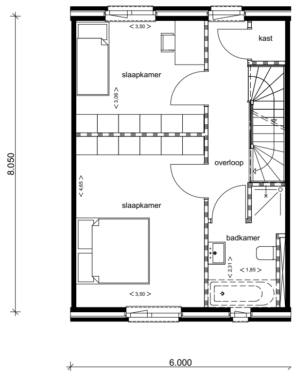
type C optie 1e verdieping kavel 1 t/m 8
