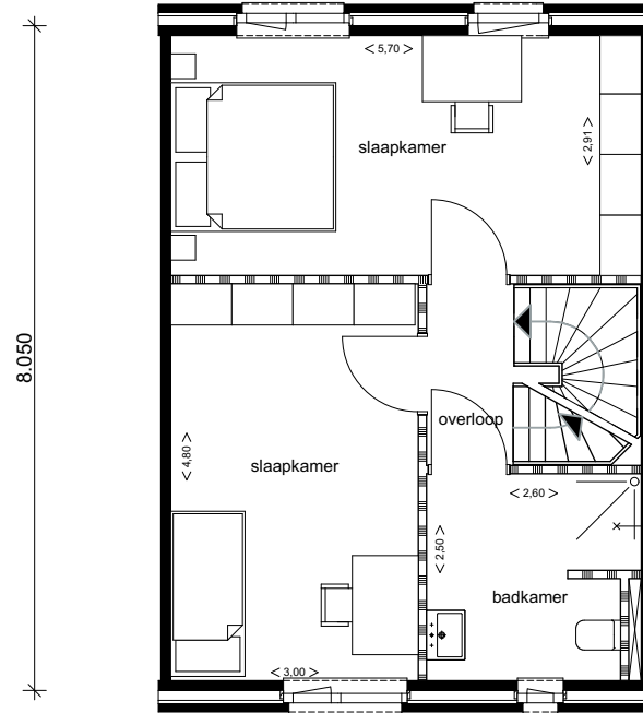
6.000 type B1 optie 1e verdieping kavel 1 t/m 8
