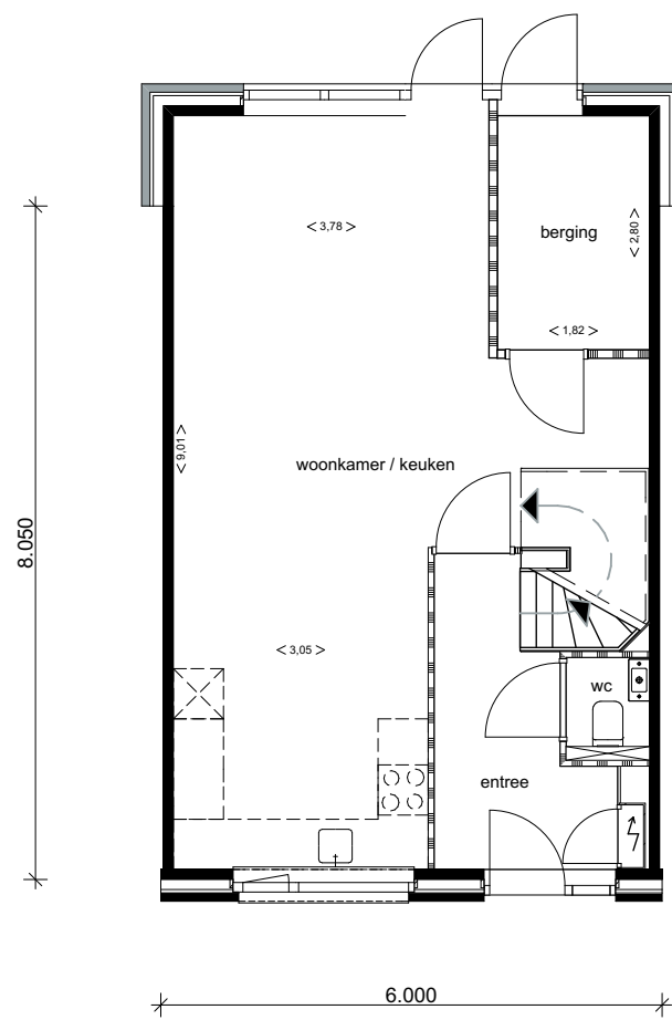
Begane grond (optie 3.2)
