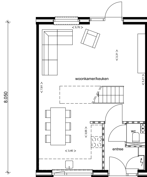
8.050 6.000 type D optie Begane grond kavel 1 t/m 8
