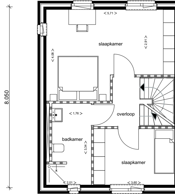
6.000 type F1 optie 1e verdieping kavel 9
