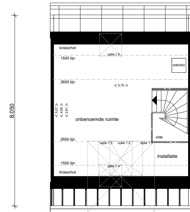
6.000 type A basis 2e verdieping kavel 1, 2, 4, 6, en 7
