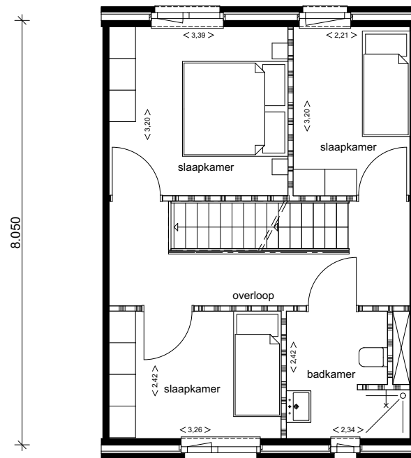
8.050 6.000 type D optie 1e verdieping kavel 1 t/m 8
