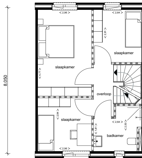
6.000 type A basis 1e verdieping kavel 1 t/m 8
