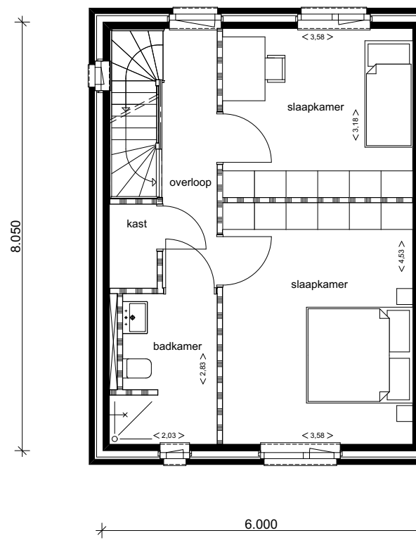
type E optie 1e verdieping kavel 9
