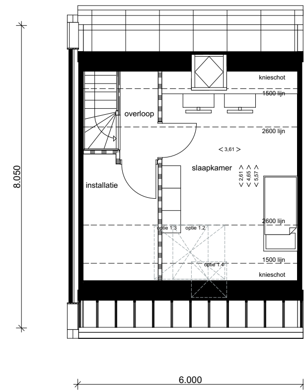
type E optie 2e verdieping kavel 9
