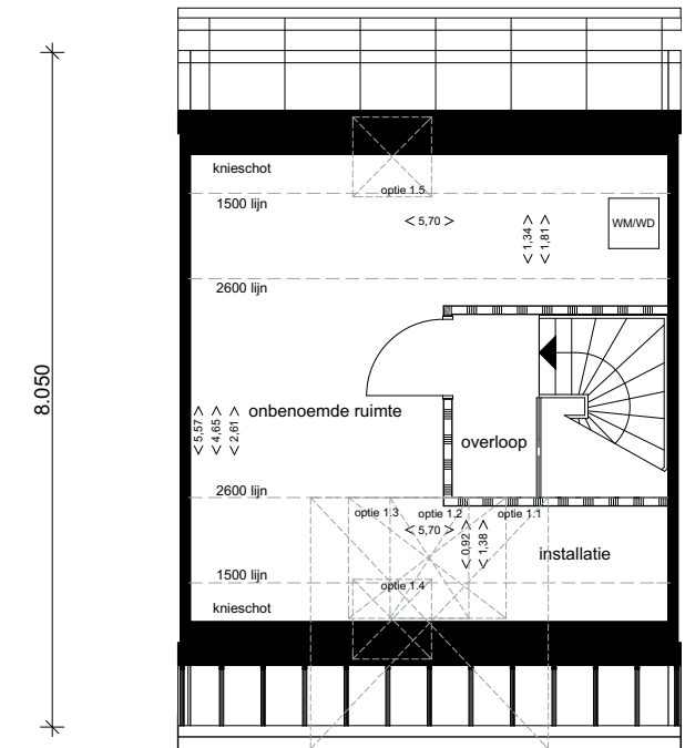
8.050 6.000 type B optie 2e verdieping kavel 1 t/m 8
