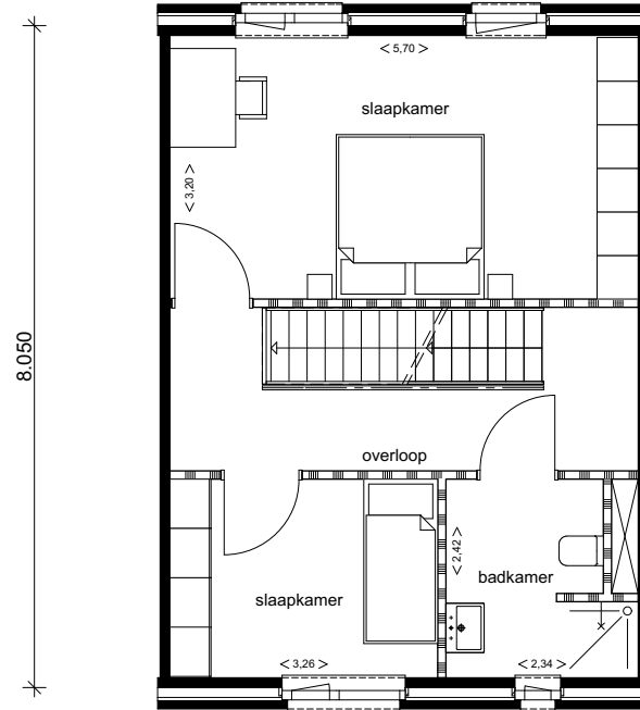
6.000 type D1 optie 1e verdieping kavel 1 t/m 8
