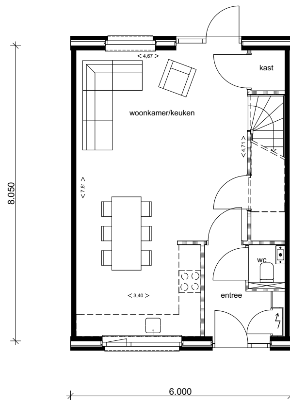
type C optie Begane grond kavel 1 t/m 8
