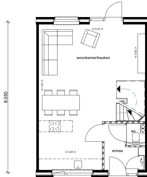
8.050 6.000 type B optie Begane grond kavel 1 t/m 8
