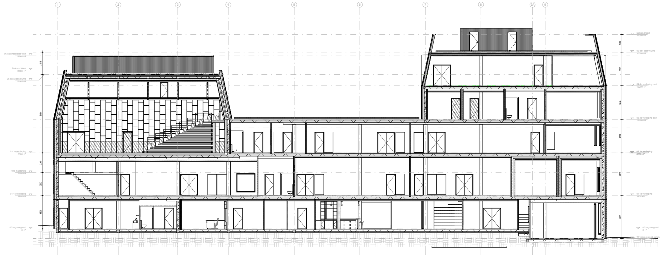
DOORSNEDE A
