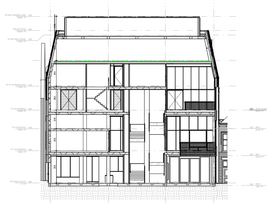
DOORSNEDE B1
