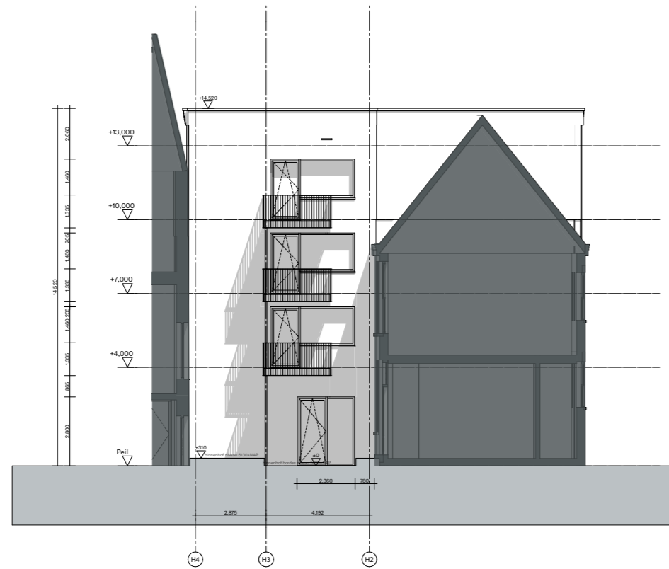
NOORDGEVEL
