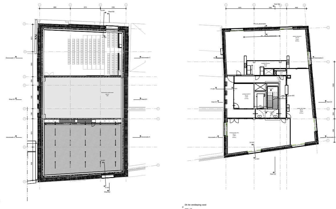
VERDIEPING 4
