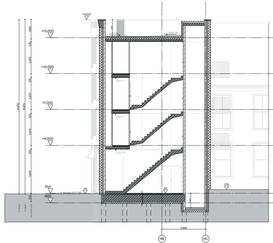
DOORSNEDE AA
