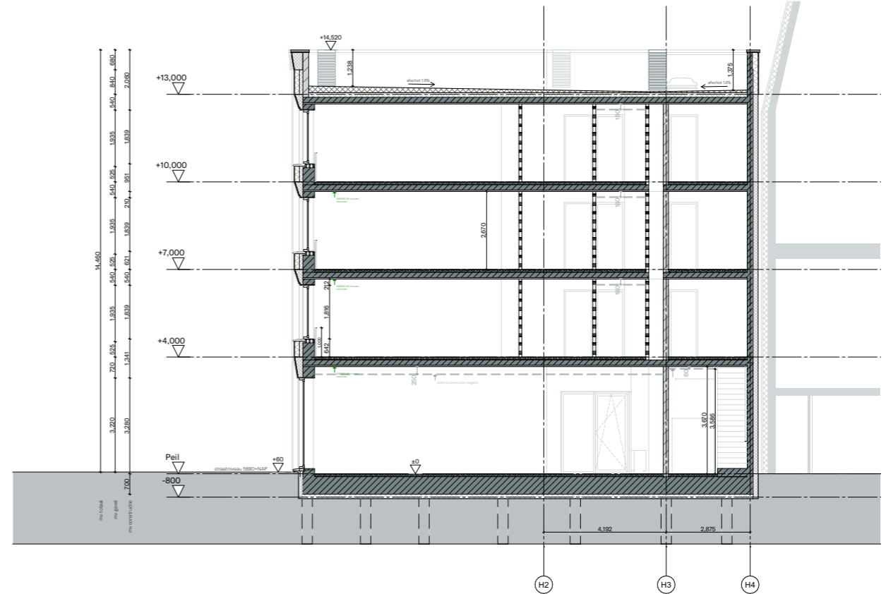
DOORSNEDE DD
