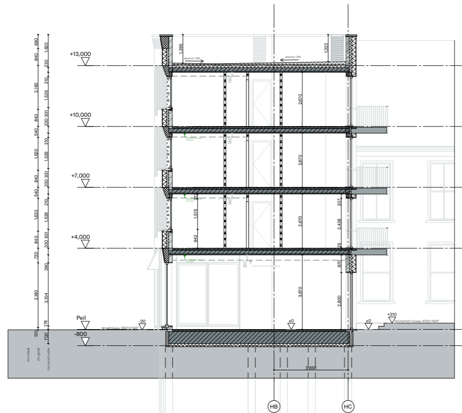
DOORSNEDE BB
