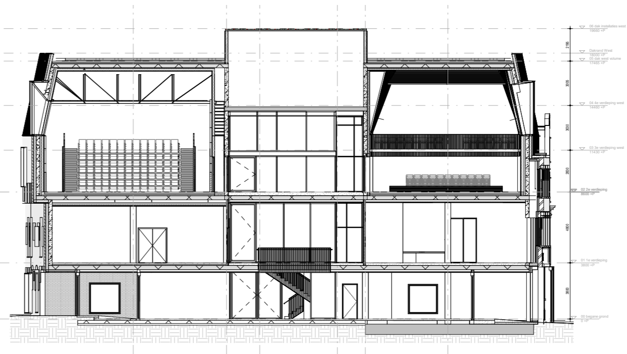
DOORSNEDE B2
