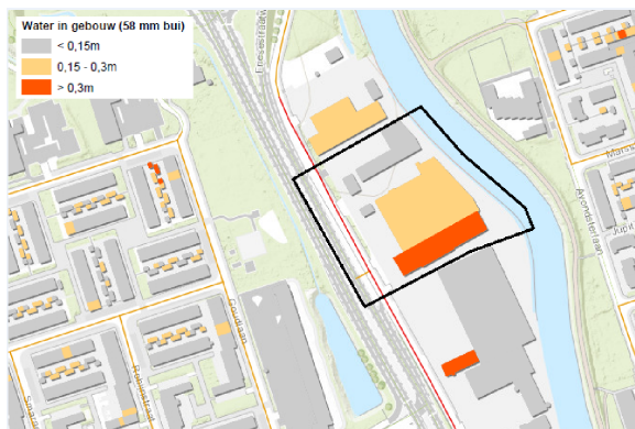
Figuur 4.5 Water in gebouw 58 mm bui
