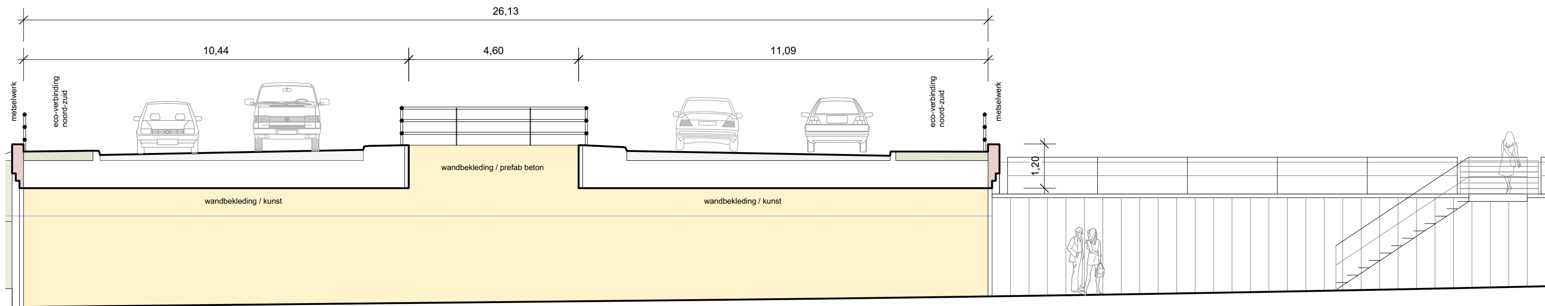
Wegviaduct / damwand
