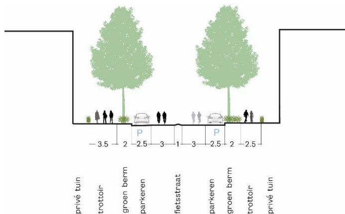
Figuur 3. Profiel Fietsstraat (t.h.v. Korreweg 228)
