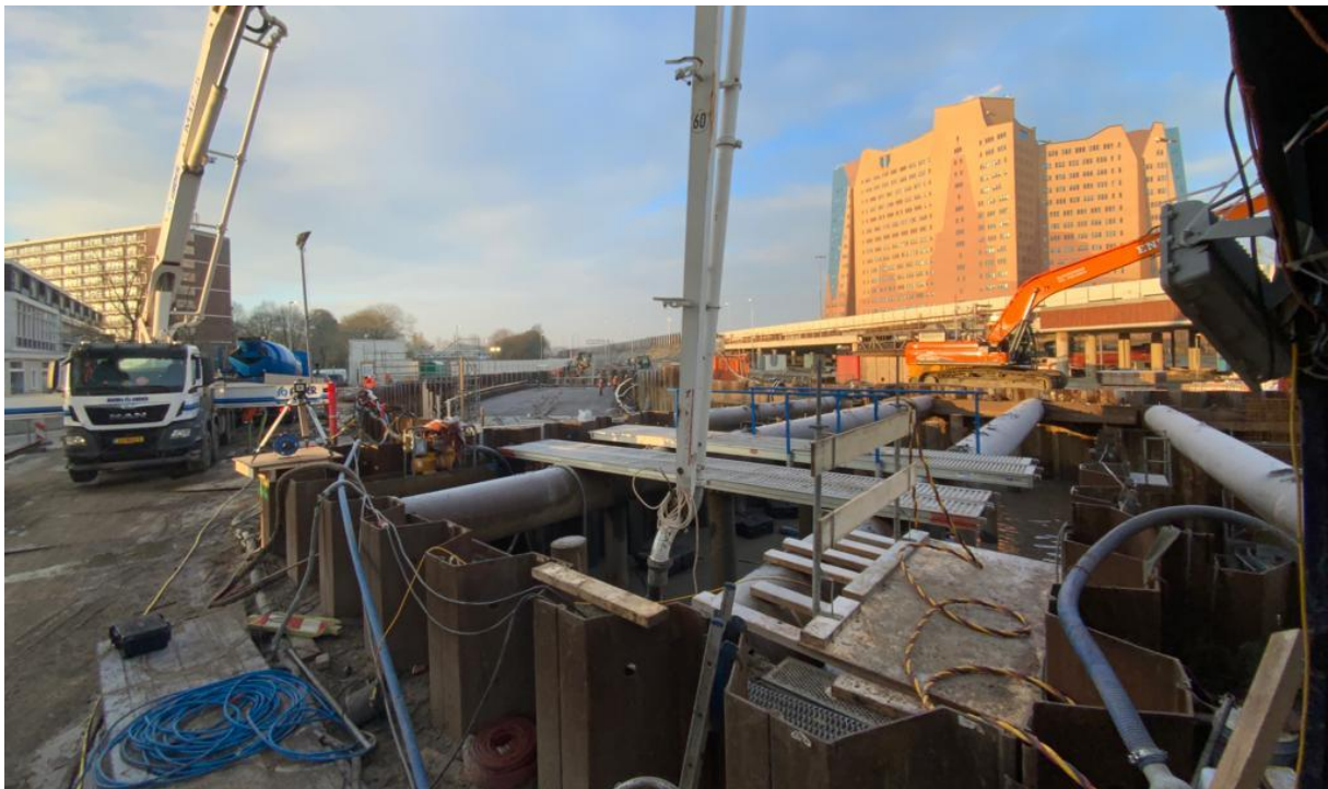
Onderwaterbetonstort Vrijheidsplein.
