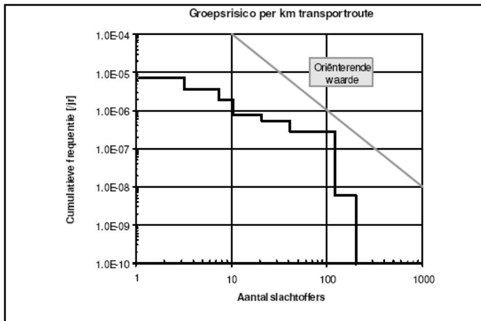
Figuur 1: Voorbeeld van een fN-curve
