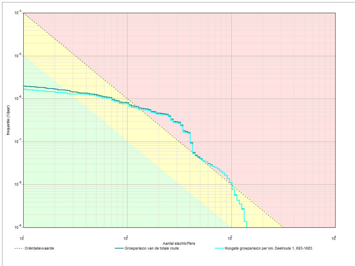
Figuur 2: Risicocurve A7
