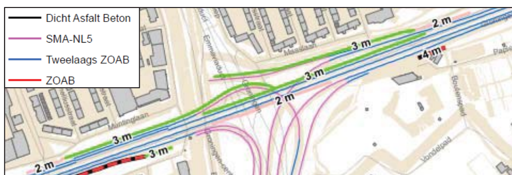
Figuur 15 Doelmatige bron- en overdrachtsmaatregelen voor het cluster Julianaplein ter plaatse van subcluster rijksweg 7 noord
