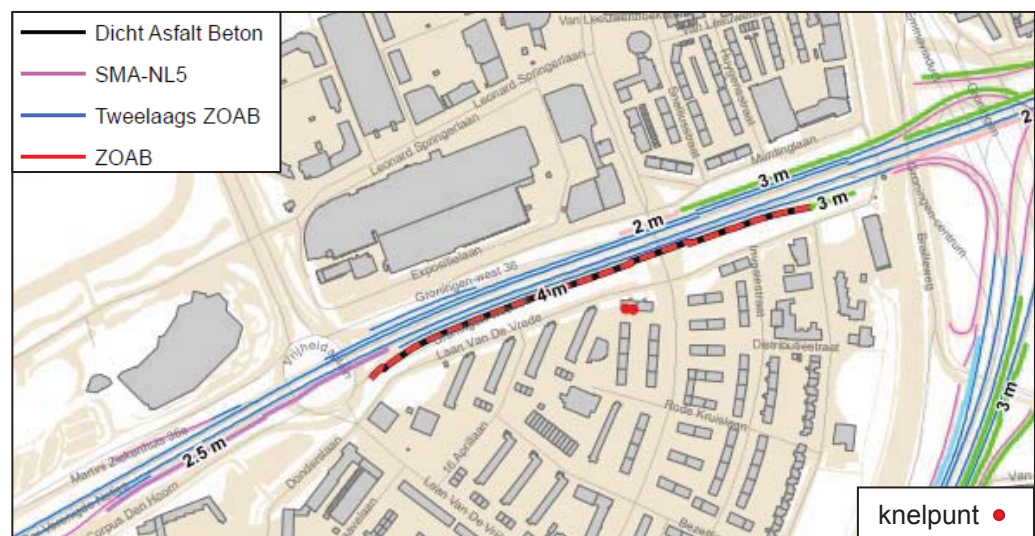
Figuur 14 Doelmatige bron- en overdrachtsmaatregelen en overgebleven knelpunten voor het cluster Julianaplein ter plaatse van subcluster rijksweg 7 west na variant SAMdoel
