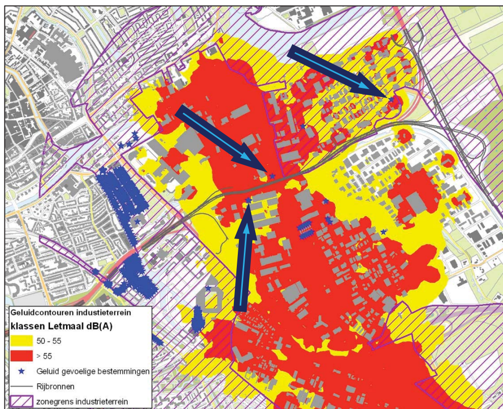
Figuur 4 Geluidzone rond het industrieterrein Groningen Zuidoost
