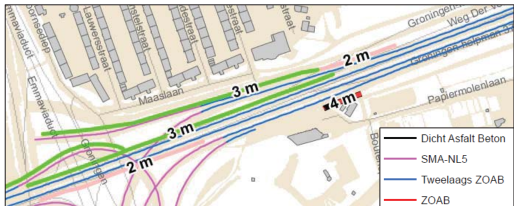
Figuur 16 Doelmatige bron- en overdrachtsmaatregelen voor het cluster Julianaplein ter plaatse van subcluster rijksweg 7 oost
