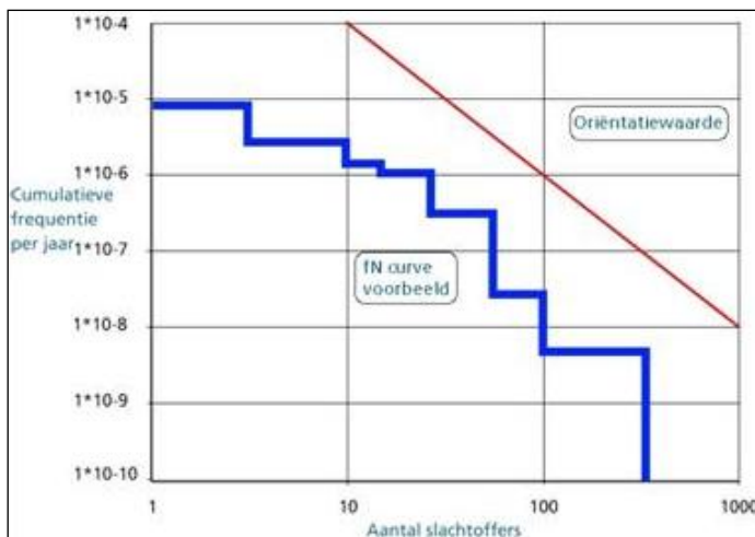
Figuur 3: Voorbeeld fN-curve
