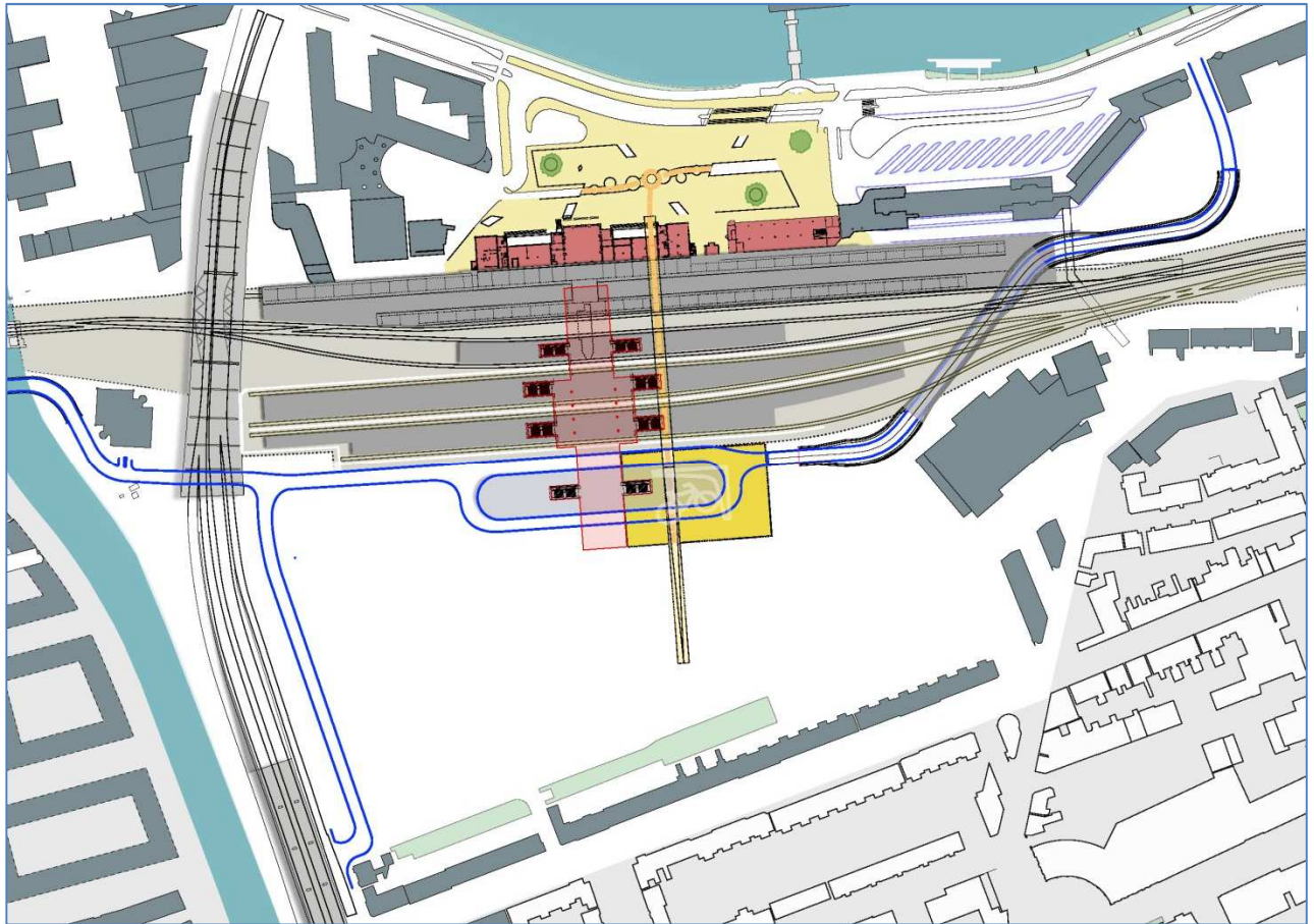
Ligging en aansluitingen bustunnel
