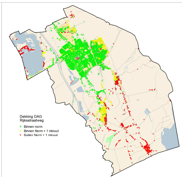
DAG SITUATIE RIJKSSTRAATWEG (TUBANTIA)
