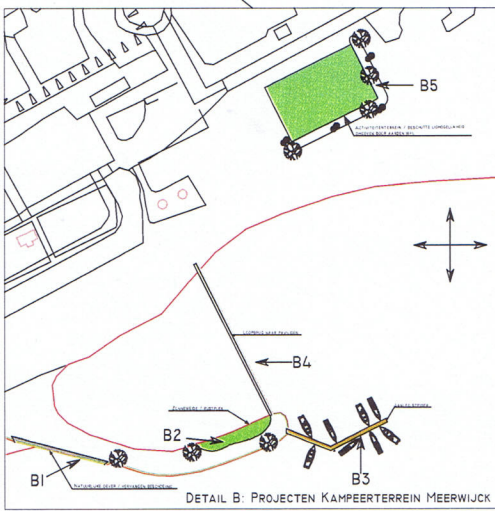
DETAIL B: PROJECTEN KAMPEERTERRAIN MEERWIJCK
