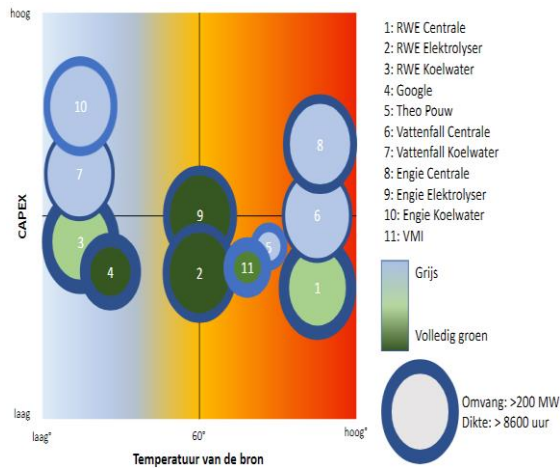
Figuur 13: Warmtebronnen
