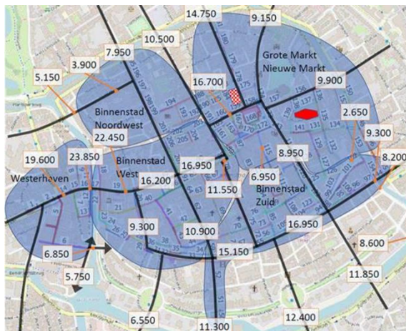
Afbeelding 2: Intensiteit fietsroutes
