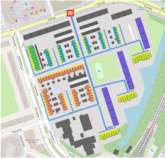
Initieel ontwerp distributienet (blauwe leidingen)
