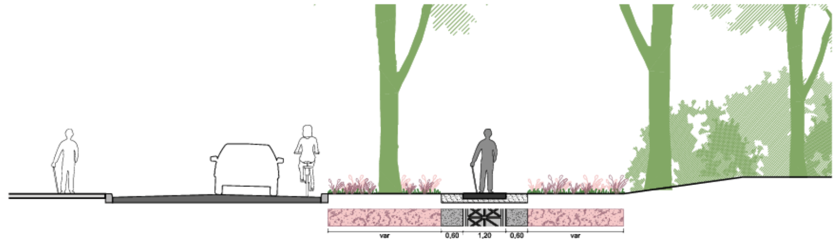
Doorsnede 2: Waterloolaan
