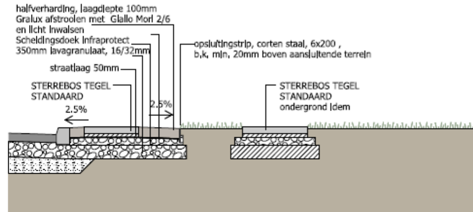
Doorsnede A-A
